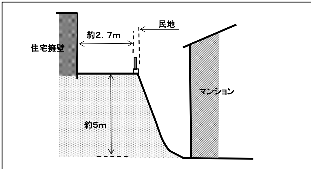
(現地概略図)
