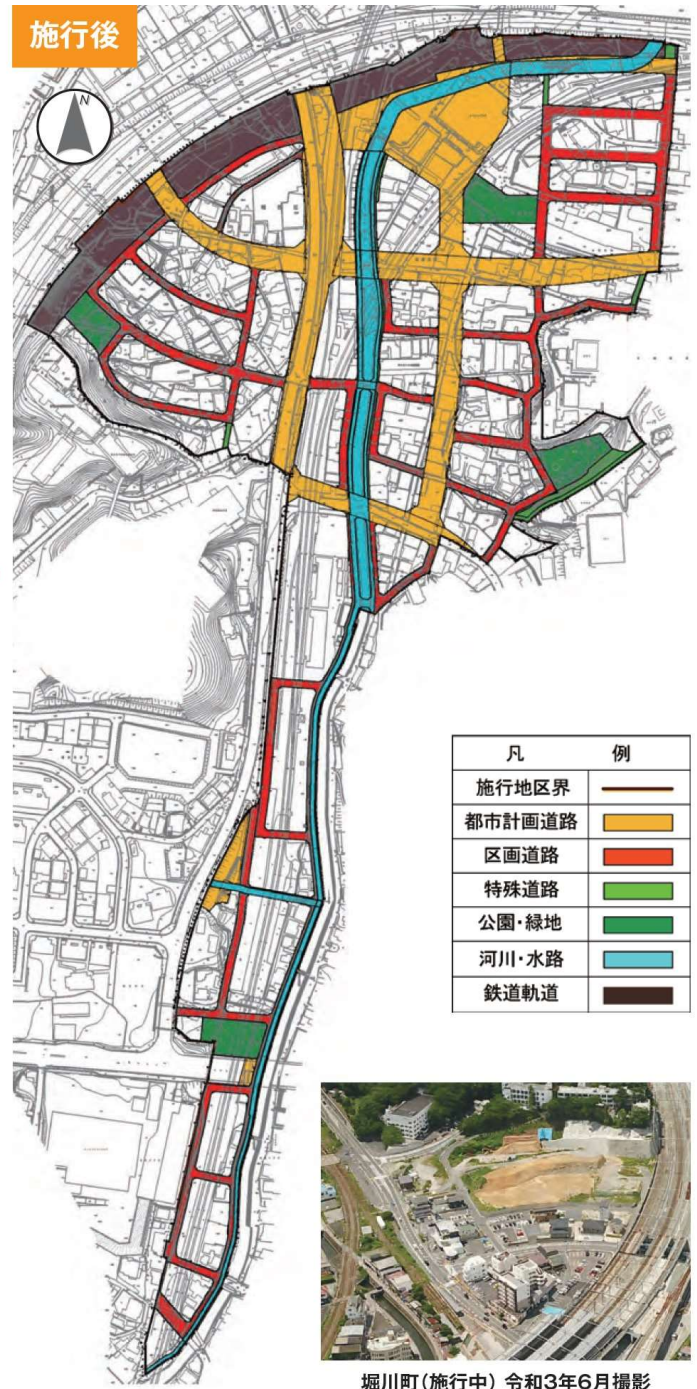
堀川町(施行中) 令和3年6月撮影
