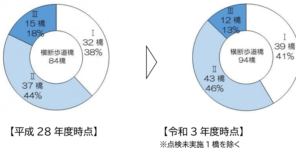
図 2.5 定期点検の結果(令和 3 年度末時点)
