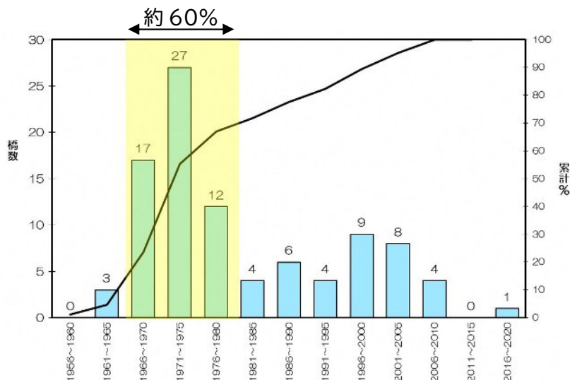
図 2.3 建設年の分布
