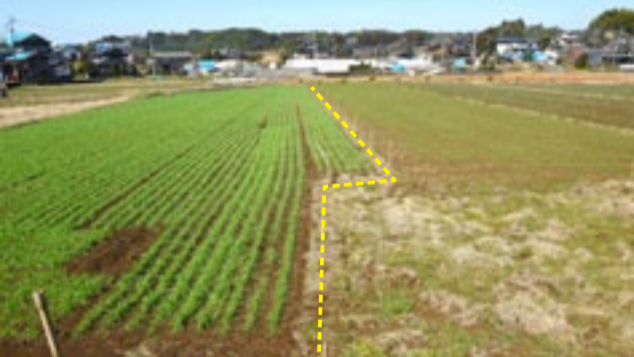
▲地震によって断層が地表に現れた場所(点線部分)。地面がずれたことがはっきりと分かる
