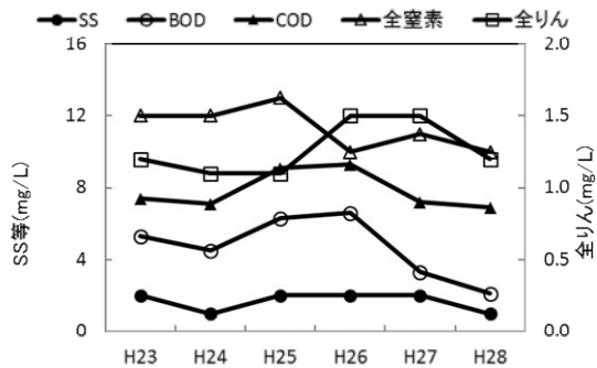
図-5 深槽処理水の経年変化
