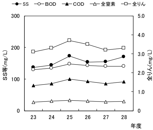
図-1 処理場流入水の経年変化
