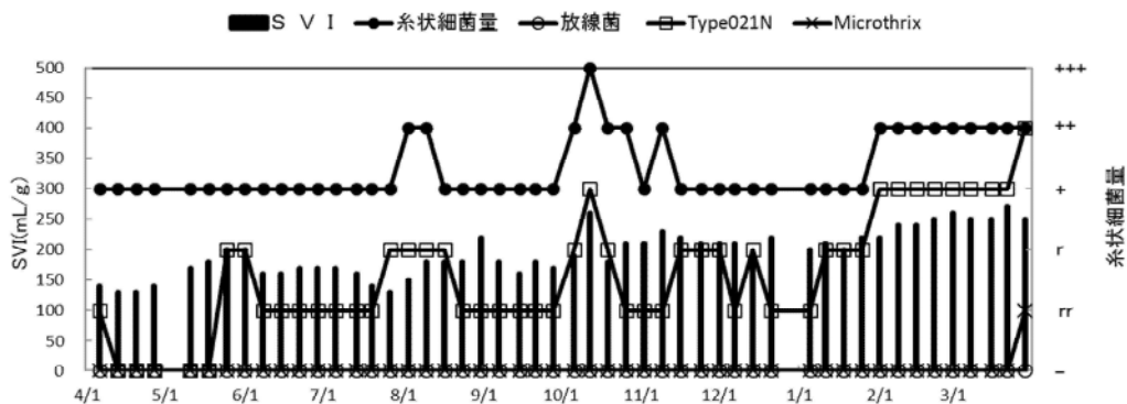
図-7 反応タンク混合液(標準槽)のSVIと糸状細菌
