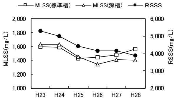
図-4 MLSS等の経年変化
