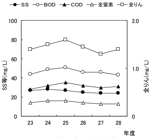
図-2 初沈流出水の経年変化
