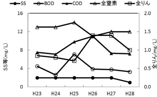
図-4 標準槽処理水の経年変化
