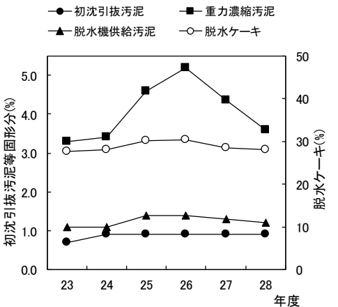
図-6 汚泥の固形分の経年変化
