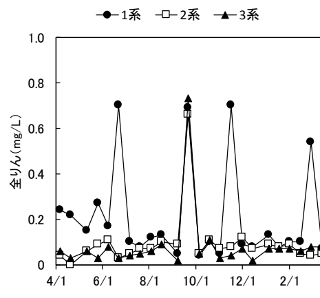
図-4 処理水中の全りん濃度変化
