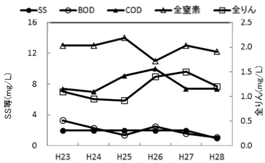
図-3 放流水の経年変化
