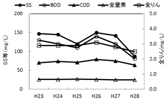
図-1 処理場流入水の経年変化
