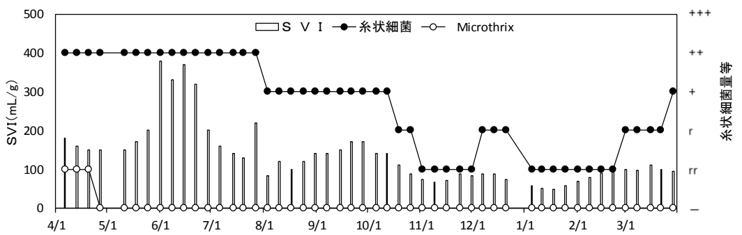
図-5 SVIと糸状細菌量の推移
