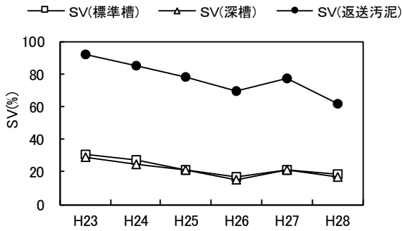
図-5 SVの経年変化
