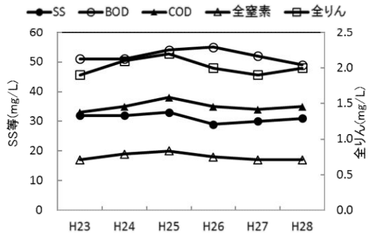
図-2 初沈流出水の経年変化
