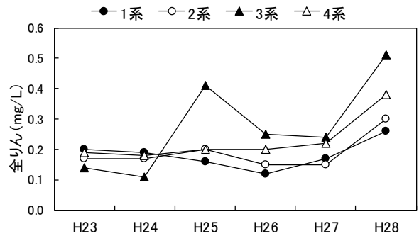
図-5 処理水の全りん径年変化
