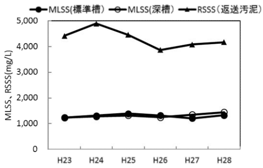
図-6 MLSS等経年変化
