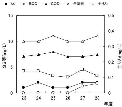
図-3 放流水の経年変化
