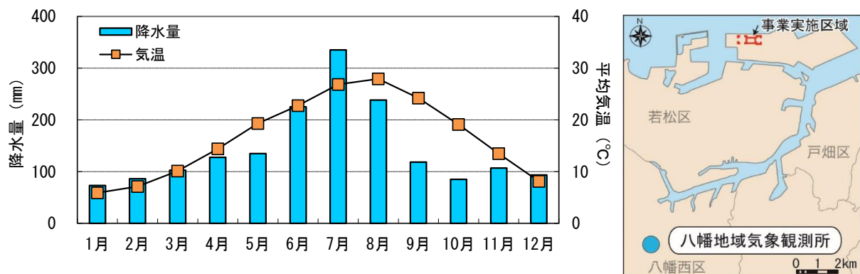
図 3-2 八幡地域気象観測所における気温と降水量（平成 18 年～27 年）
