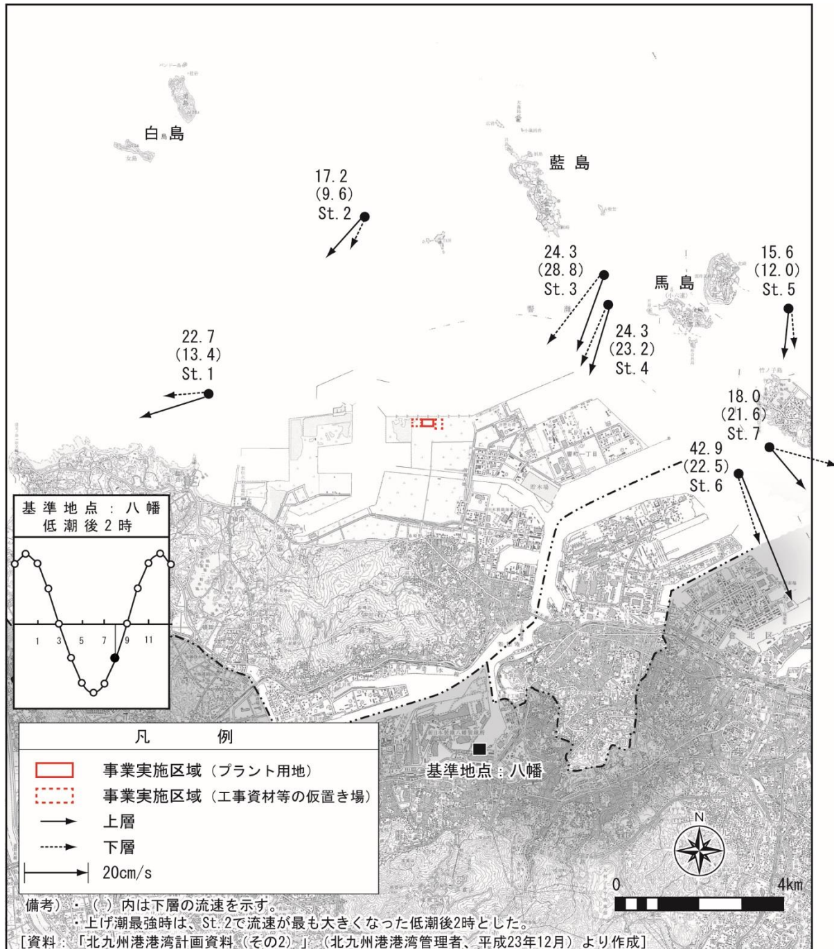
図 3-10 平均大潮期の流況（上げ潮最強時）
