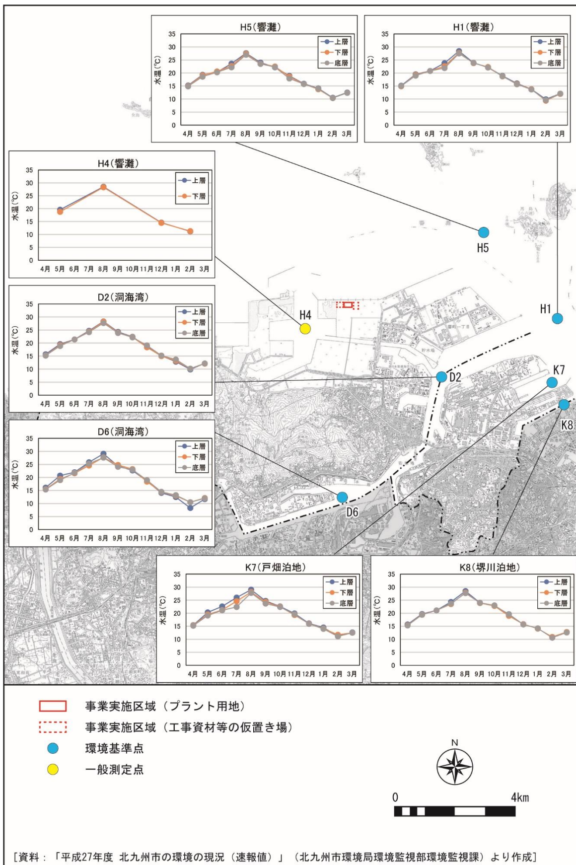
図 3-17 海域における水温の経月変化
