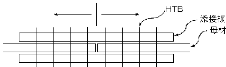
図2-1 ボルト締め付け順序
