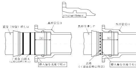
図3-7-37 挿入量の明示
