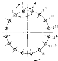
図3-7-4 追い締め付け
