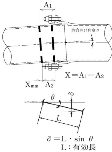
図3-7-5 曲げ角度と偏位
