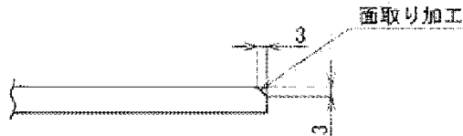
図 3-7-49 挿し口の面取り
