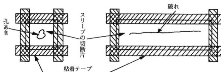
図 3-6-4 スリーブの補修
