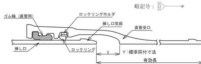
図3-7-38 直管の継手構造
