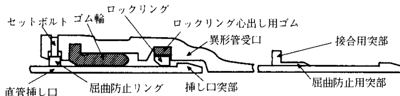
図3-7-13 異形管の継手構造(呼び径75～250)
