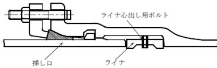
図3-7-23 直管の継手構造（ライナ使用）
