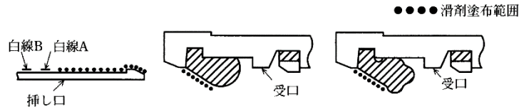
図3-7-8 滑剤塗布範囲
