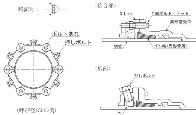
図3-7-54 G - Linkの構造
