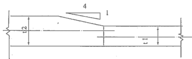
図 3-8-3 管厚の異なる溶接継手
