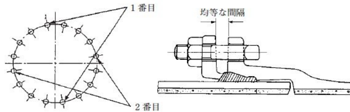
図3-7-3 仮締め付け
