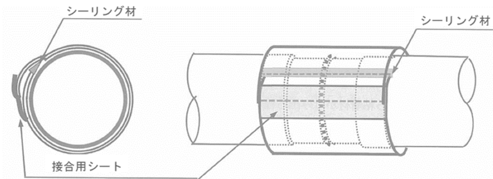
図 3-8-6 熱収縮シート巻き終わり部の施工
