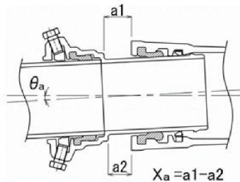
図 3-7-53 曲げ角度確認方法
