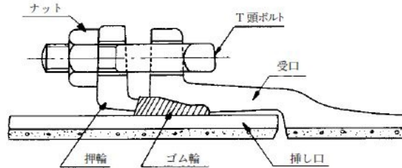
図3-7-1 継手構造
