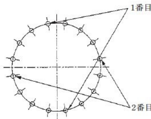
図3-7-56 仮締め付け
