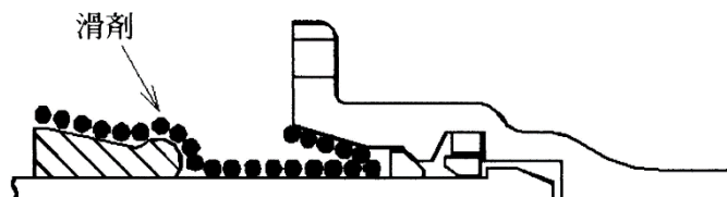
図3-7-19 滑剤塗布範囲
