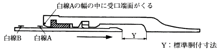
図3-7-9 挿入状態
