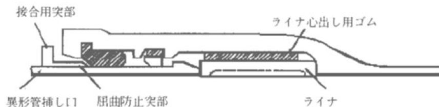
図3-7-7 直管の継手構造(呼び径75～450ライナ使用)
