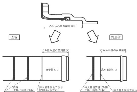
図3-7-46 挿し口挿入量の明示
