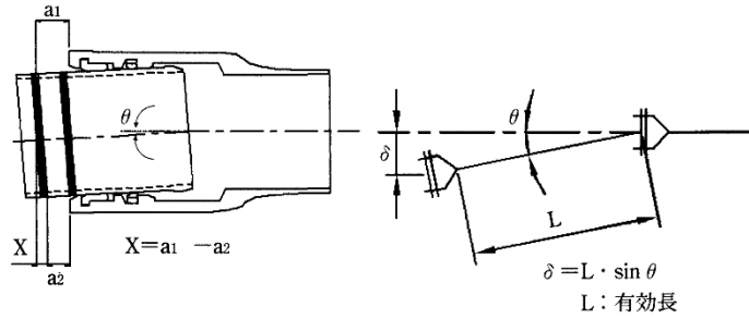
図 3-7-12 曲げ角度と偏位
