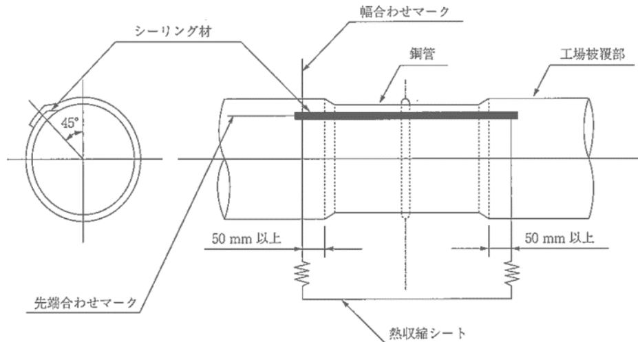
図 3-8-5 熱収縮シートの巻付け
