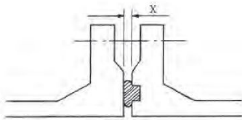
図3-7-58 X寸法
