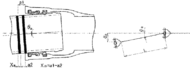
図 3-7-44 曲げ角度と偏位
