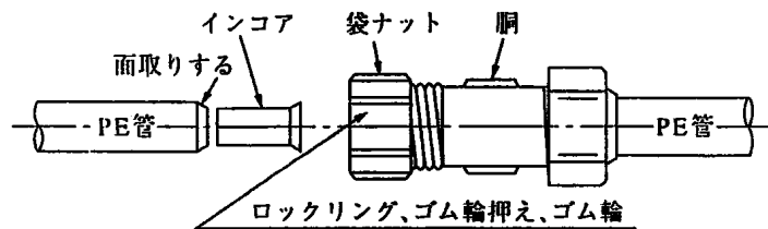
図3-6-1 冷間接合A形
