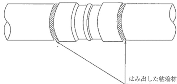
図 3-8-8 施工確認
