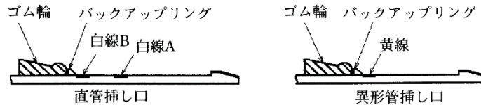
図3-7-18 接合部品のセット位置
