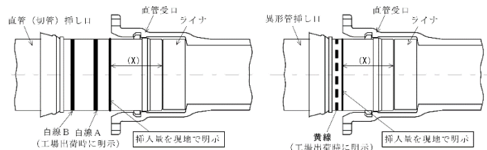
図3-7-28 挿入量の明示
