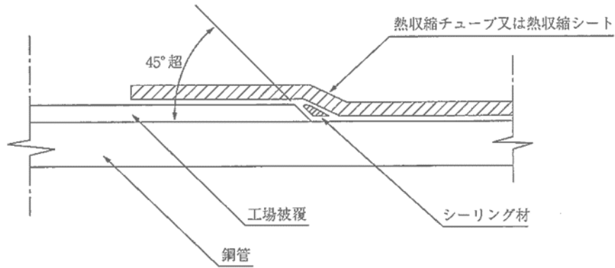
図 3-8-4 シーリング材の施工
