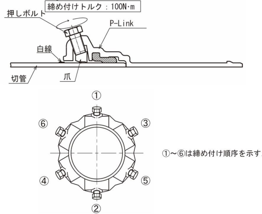
図 3-7-51 押しボルトの締め付け
