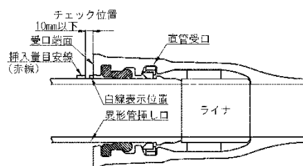
図3-7-43 异形管挿し口(P Link)を接合する場合のチェック位置と白線表示位置
