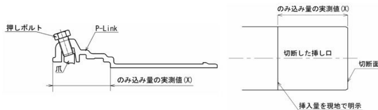
図 3-7-50 挿し口挿入量の明示
