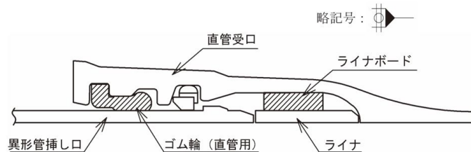
図3-7-39 直管の継手構造 (ライナ使用)
