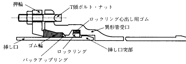
図3-7-15 異形管の継手構造(呼び径300~450)
