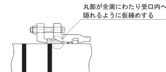
図3-7-31 仮締めとゴム輪の押し込み
