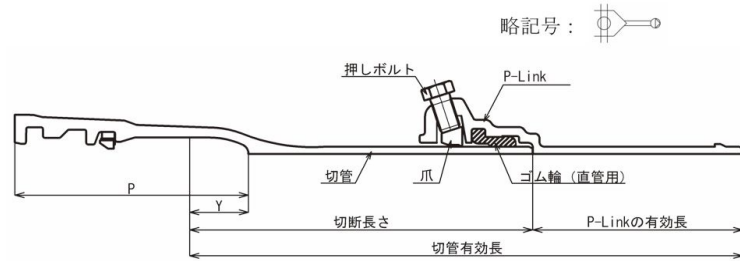
図3-7-48 P - L i n k の構造
