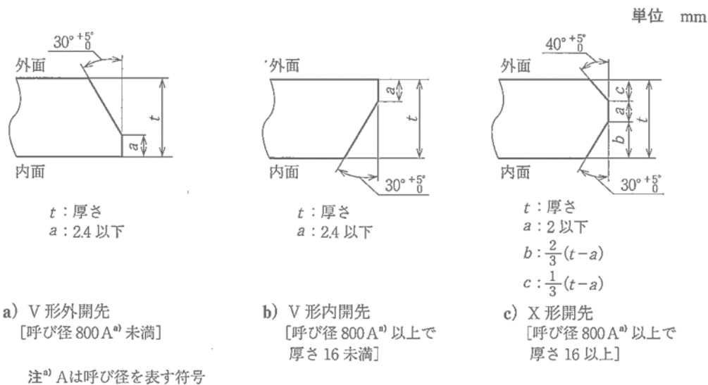
図 3-8-1 開先形状
