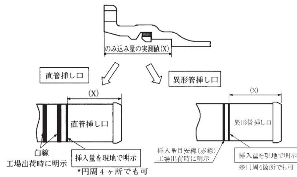
図3-7-16 挿し口の挿入量
