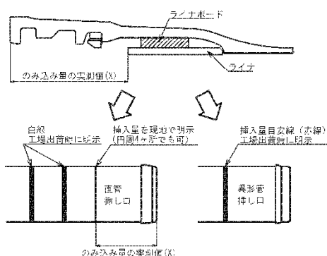
図3-7-42 挿し口挿入量の明示
