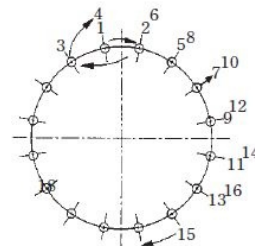
3-7-57 追い締め付け
