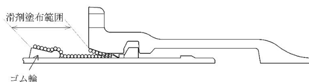
図3-7-30 滑剤塗布範囲
