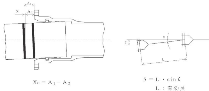
図3-7-33 許容曲げ角度と偏位
