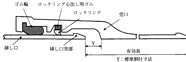
図3-7-6 直管の継手構造(呼び径75～450)
