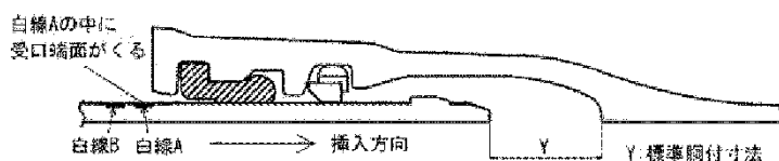
図3-7-41 挿入状態
