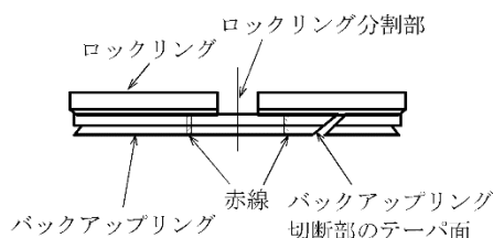
図3-7-29 バックアップリング切断部の確認
