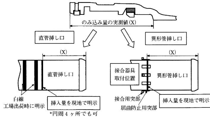
図3-7-14 挿し口挿入量
