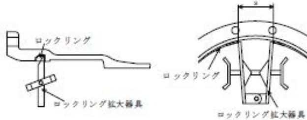
図3-7-25 ロックリング拡大器具の装着
