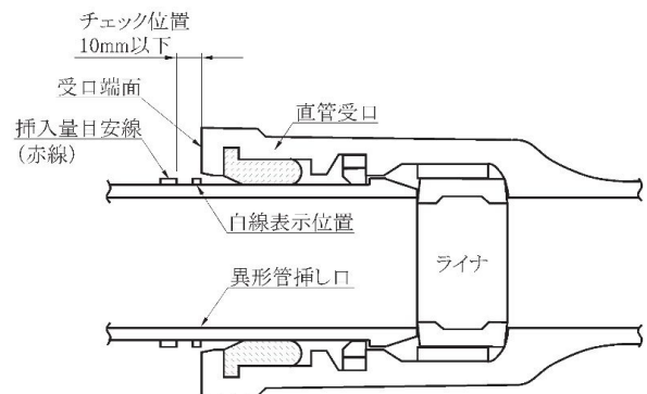
図3-7-11 異形管挿し口(呼び径300~450)を接合する場合のチェック位置と白線表示位置
