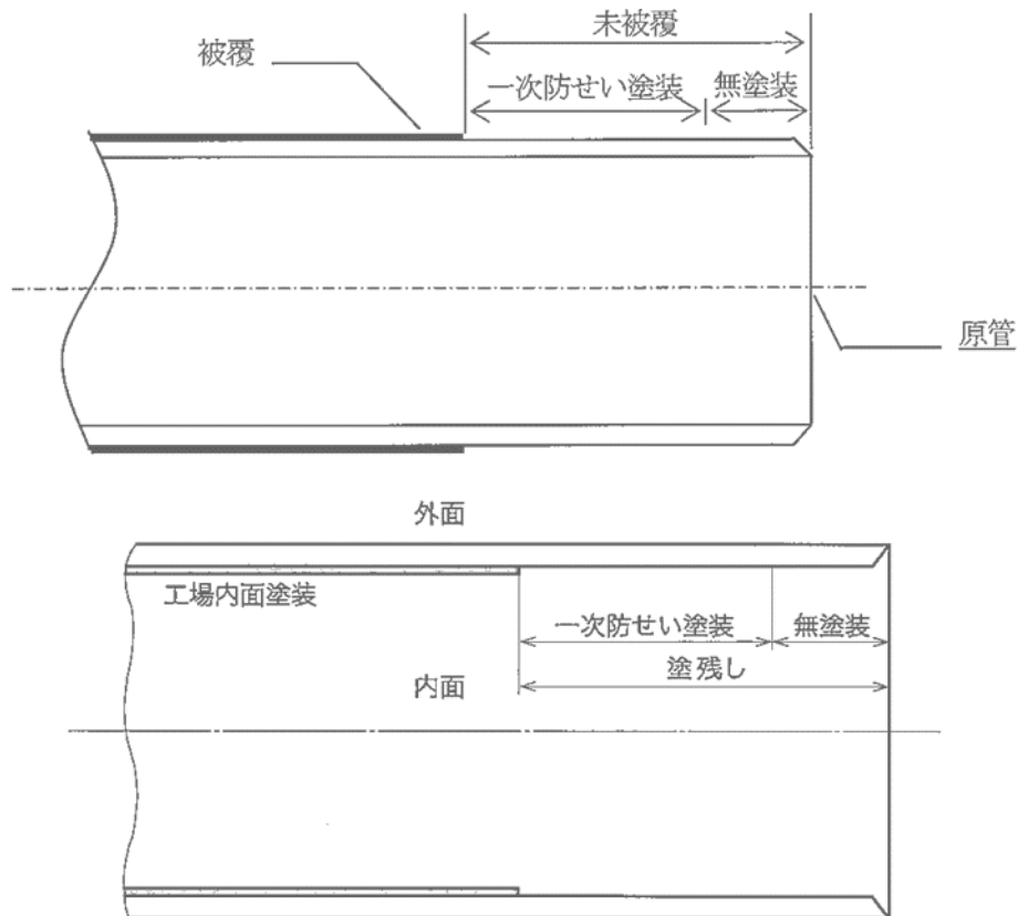
図 3-8-2 管端未被覆長さ
