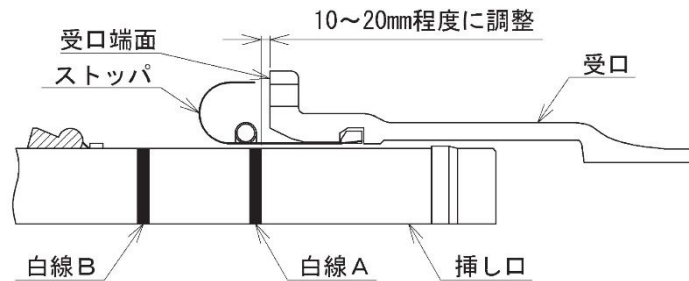
図3-7-27 挿し口の挿入
