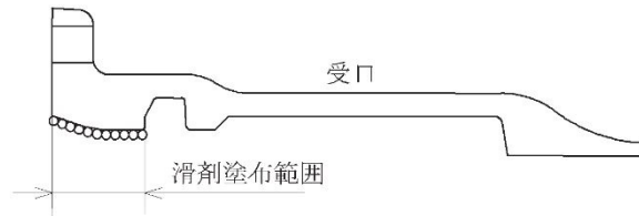
図3-7-26 滑剤塗布範囲
