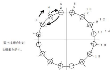
図3-7-34 追い締め付け方法
