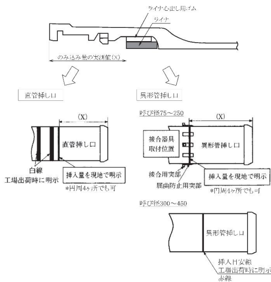
図3-7-10 挿し口挿入量の明示
