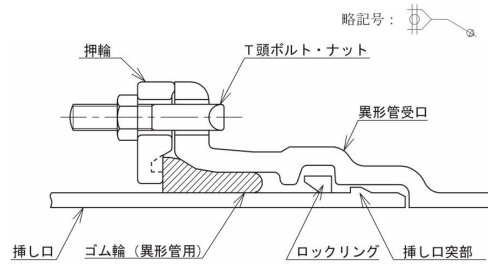
図 3-7-45 異形管の継手構造
