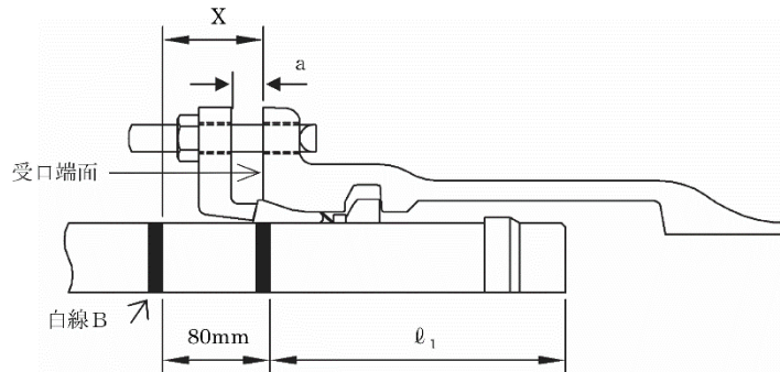
図3-7-35 受口端面と押輪間隔および受口端面と白線間隔の計測 チェックシートへの記入は、接合作業の都度行う。
