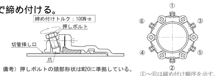
図3-7-55 押しボルトの締め付け
