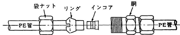
図3-6-2 冷間接合B形
