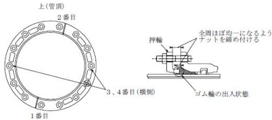
図3-7-32 ボルト・ナットの締め付け
