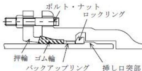
図3-7-36 異形管の継手構造(呼び径500~1000)
