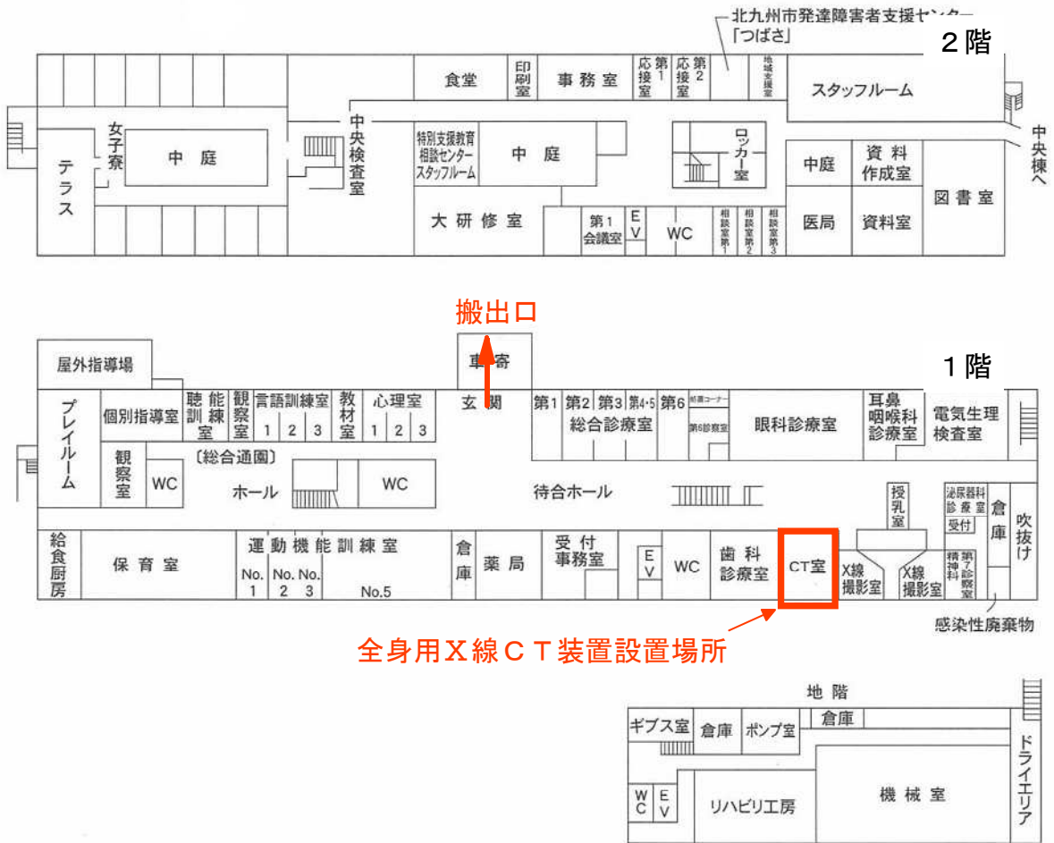
① 西 棟 平 面 図 (昭和53年10月竣工)
