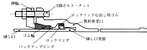
図3-7-15 異形管の継手構造(呼び径300~450)
