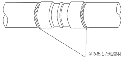
図 3-8-8 施工確認
