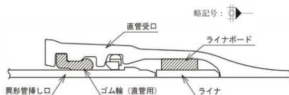
図3-7-39 直管の継手構造 (ライナ使用)
