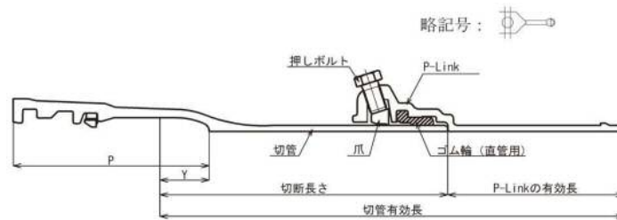
図3-7-48 P-Linkの構造
