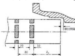
図3-7-2 接合図
