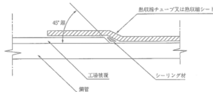
図 3-8-4 シーリング材の施工
