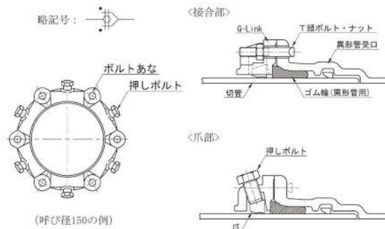
図3-7-54 G—Linkの構造
