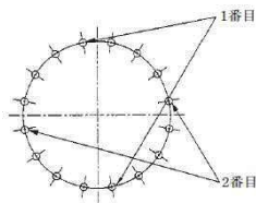
図3-7-56 仮締め付け
