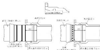
図3-7-37 挿入量の明示
