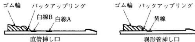
図3-7-18 接合部品のセット位置
