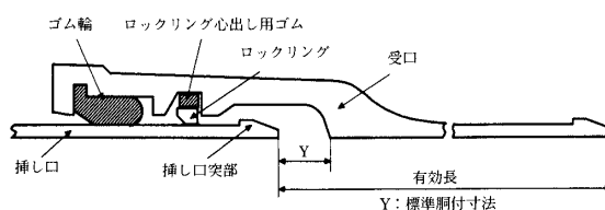
図3-7-6 直管の継手構造(呼び径75~450)
