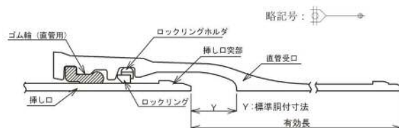
図3-7-38 直管の継手構造
