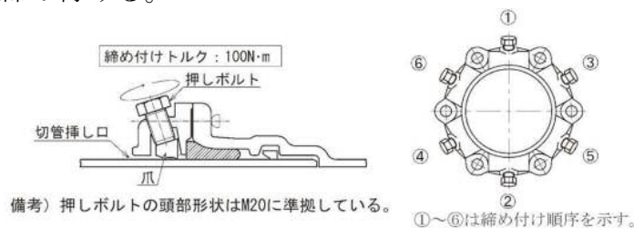
図3-7-55 押しボルトの締め付け
