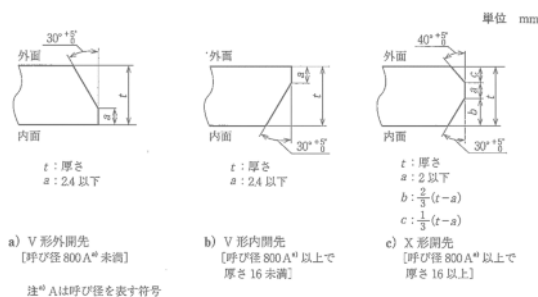
図 3-8-1 開先形状
