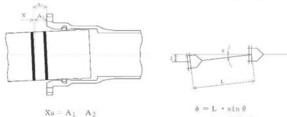
図3-7-33 許容曲げ角度と偏位
