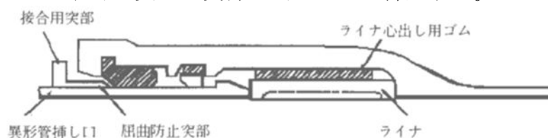
図3-7-7 直管の継手構造(呼び径75~450ライナ使用)
