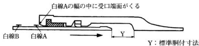
図3-7-9 挿入状態
