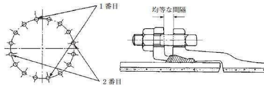
図3-7-3 仮締め付け
