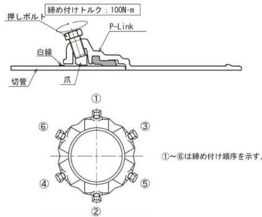
図 3-7-51 押しボルトの締め付け
