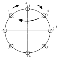
図3-7-20 追い締め付け
