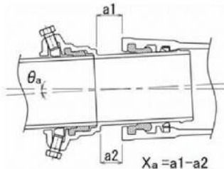
図 3-7-53 曲げ角度確認方法
