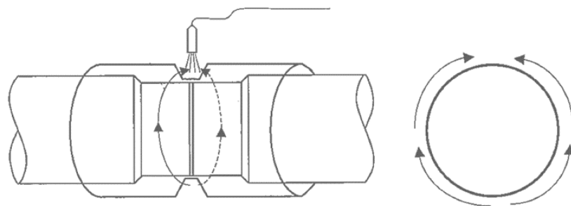
図 3-8-7 熱収縮シートの加熱
