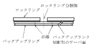
図3-7-29 バックアップリング切断部の確認
