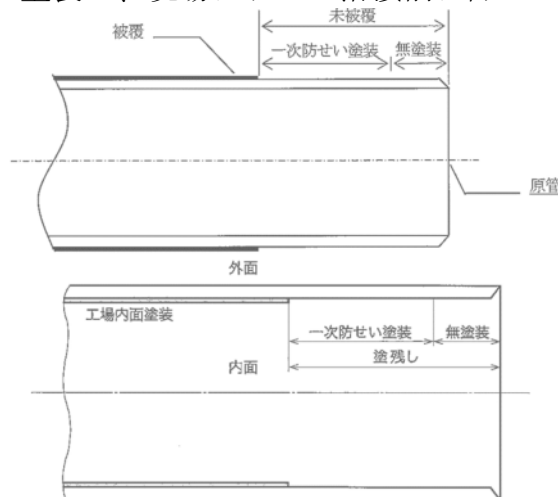
図3-8-2 管端未被覆長さ
