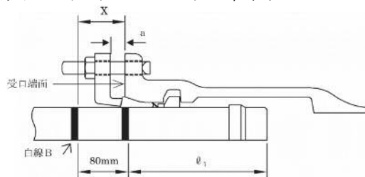
図3-7-35 受口端面と押輪間隔および受口端面と白線間隔の計測
