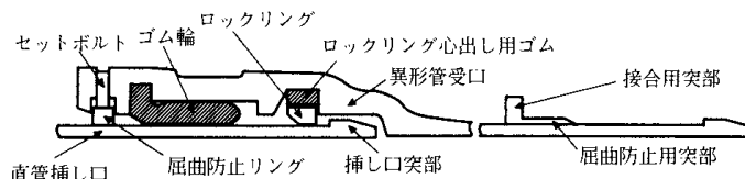
図3-7-13 異形管の継手構造(呼び径75~250)
