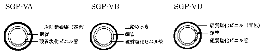
図6-2 硬質塩化ビニルライニング鋼管 (参考)
