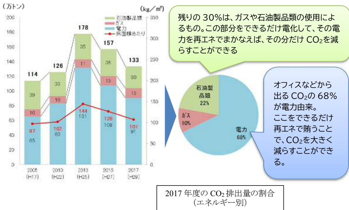
図表 6-7 CO 2 排出量の推移(業務部門)
