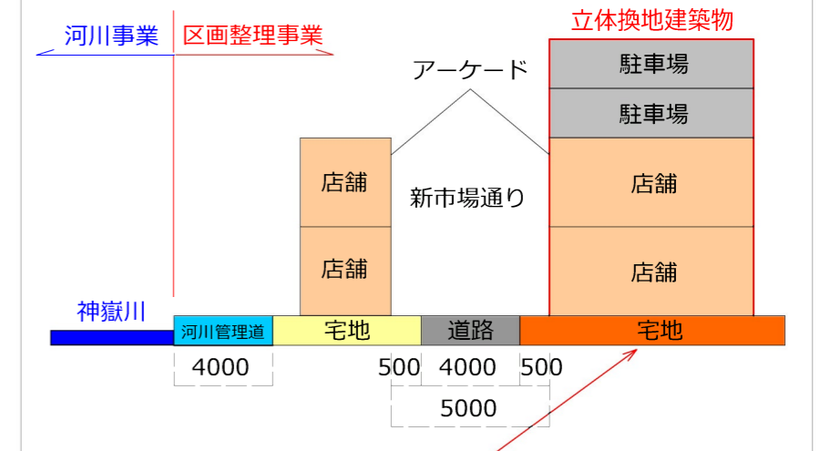
【計画断面図】
