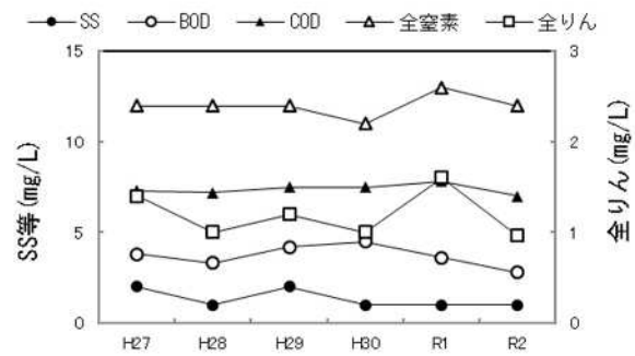
図-4 標準槽処理水の経年変化
