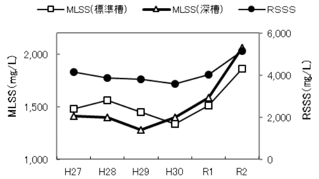
図-4 MLSS等の経年変化
