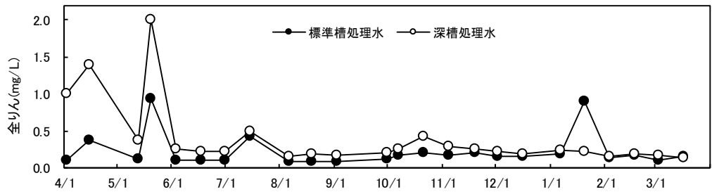
図-5 処理水の全りん濃度
