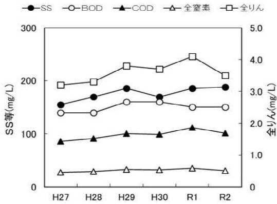
図-1 処理場流入水の経年変化
