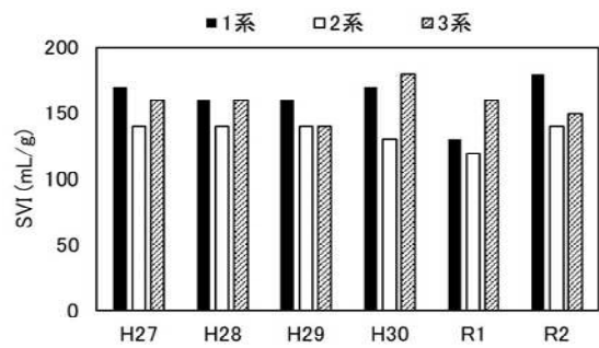
図-7 SVIの経年変化
