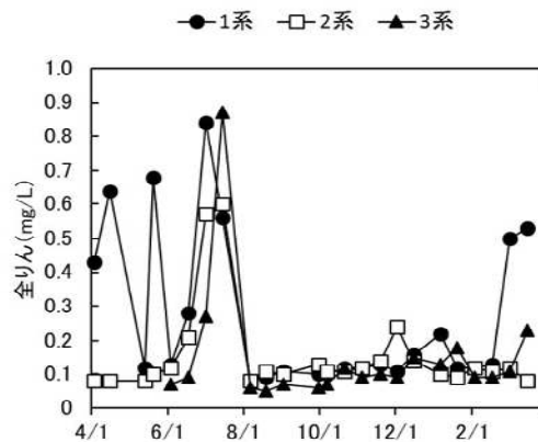
図-4 処理水中の全りん濃度変化
