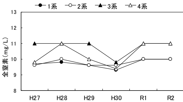
図-4 処理水の全窒素の経年変化
