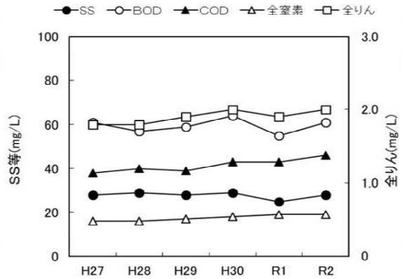
図-2 初沈流出水の経年変化
