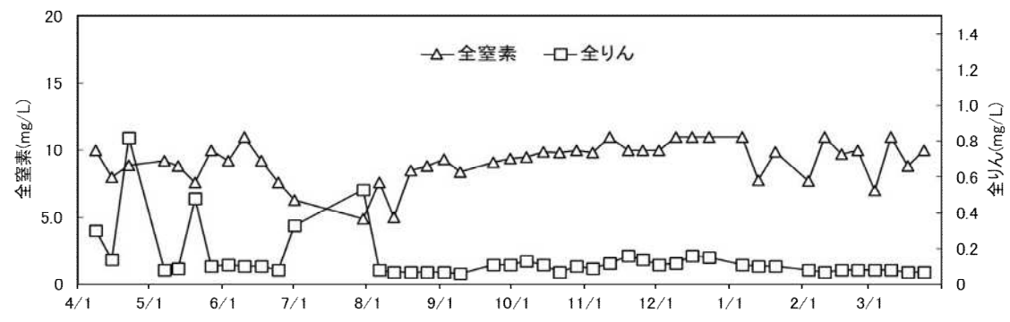
図-4 放流水中の全窒素と全リンの濃度変化
