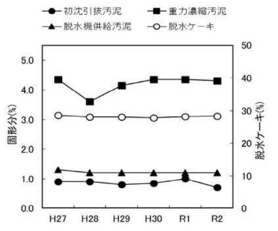
図-6 汚泥の固形分の経年変化
