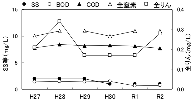
図-3 放流水の経年変化
