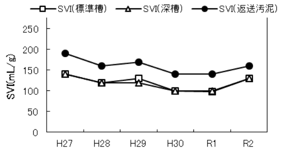
図-6 SVIの経年変化
