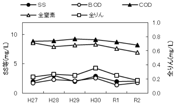
図-3 放流水の経年変化
