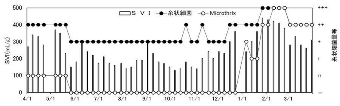
図-5 SVIと糸状細菌量の推移
