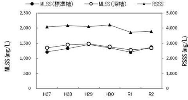
図-6 MLSS等経年変化
