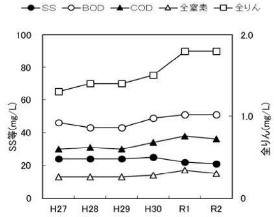
図-2 初沈流出水の経年変化
