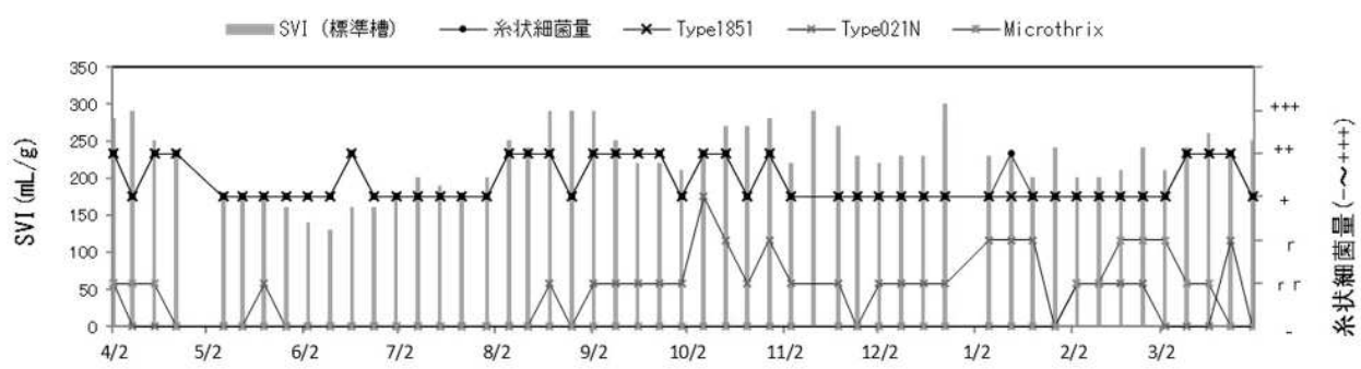
図-7 反応タンク混合液(標準槽)のSVIと糸状細菌
