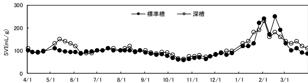
図-6 反応タンク混合液のSVI
