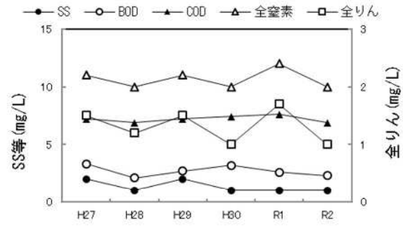
図-5 深槽処理水の経年変化
