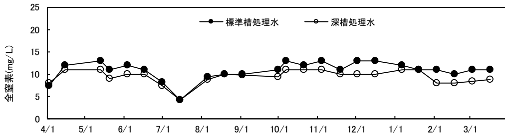
図-4 処理水の全窒素濃度
