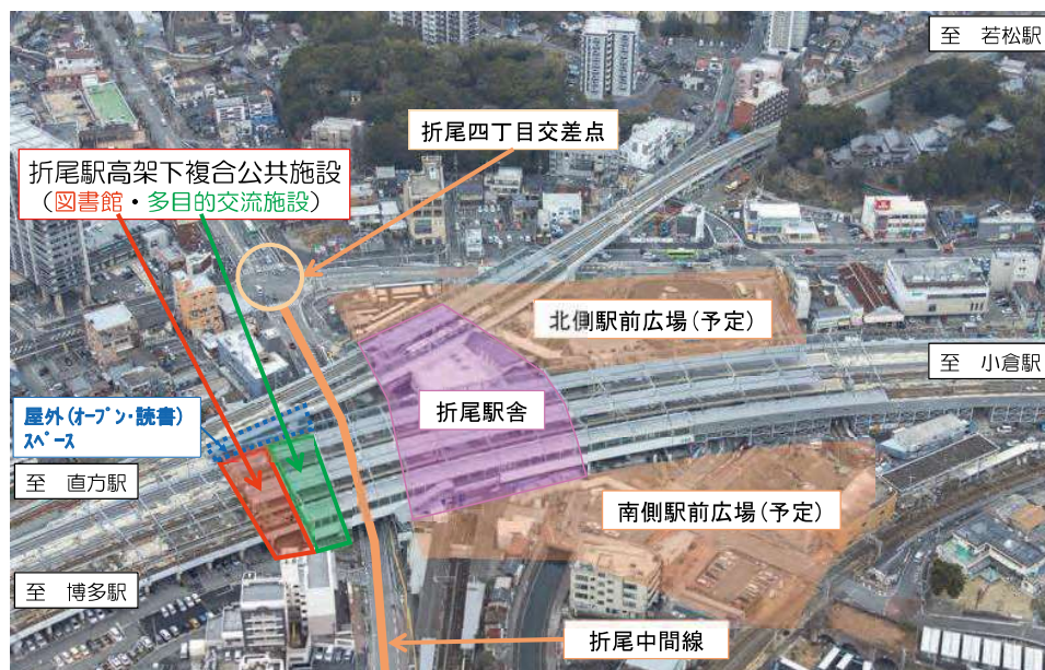
整備イメージ（外観パース）
