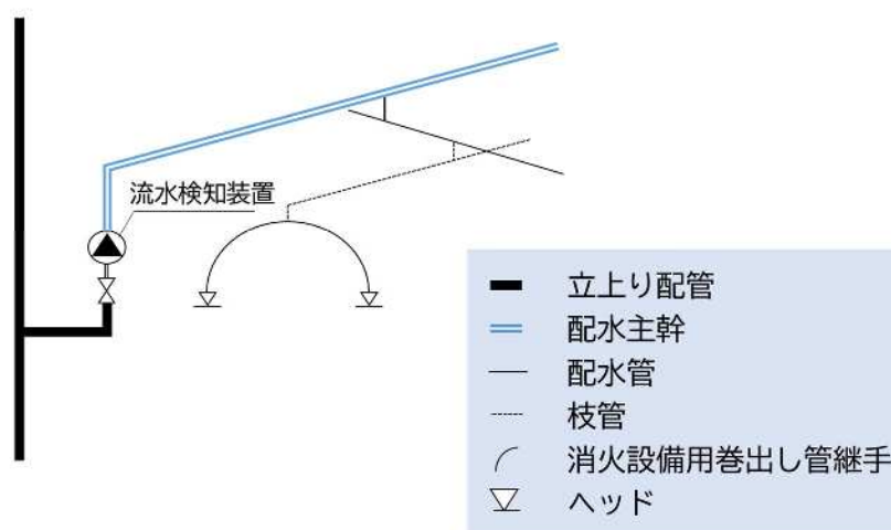
(配水管、枝管等の構成例)
