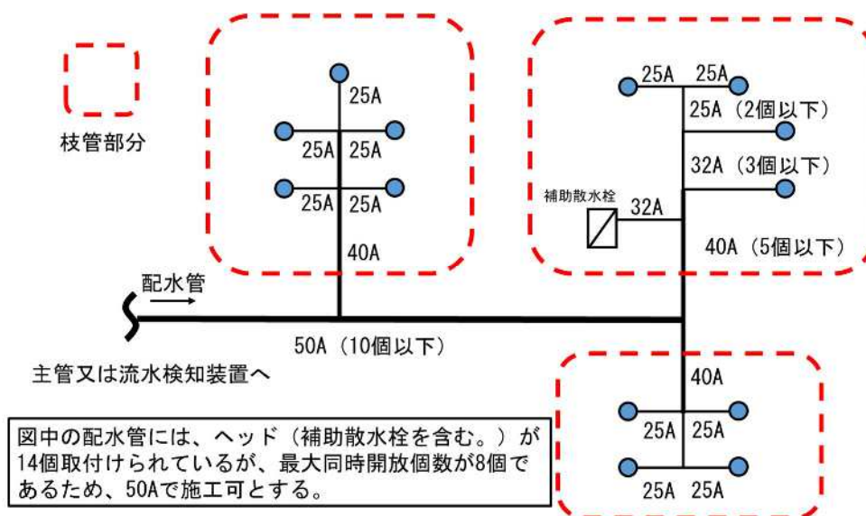
第4-4図 配置の設置例：標準型ヘッド（最大同時開放個数8個）の場合
