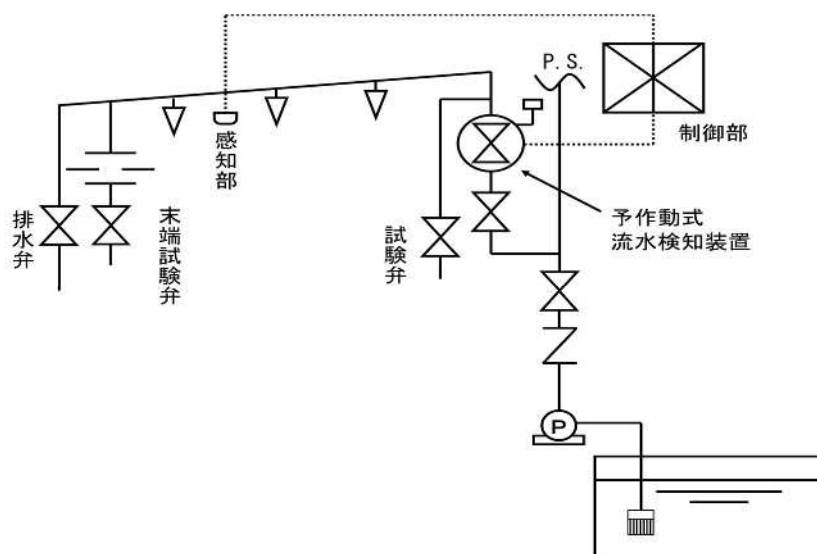
第4-31図 予作動式流水検知装置の場合
