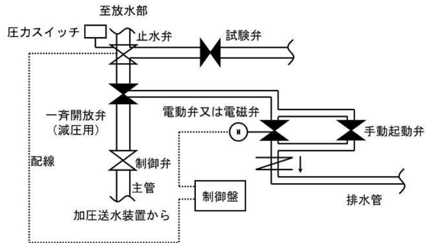
第4-17 図（減圧方式の一斉開放弁等の廻りの配管図例）
