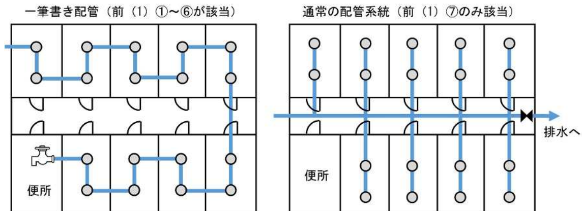
第4-40 図 一筆書き配管の例
