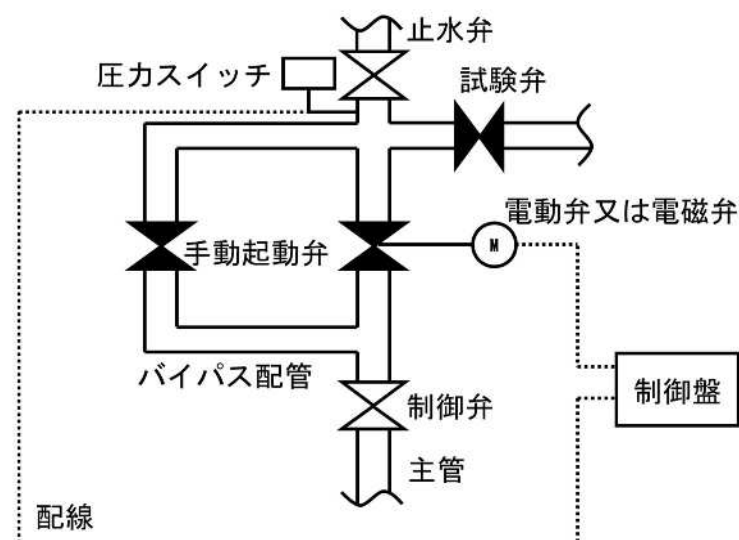
第4-19 図（電動又は電磁弁方式の廻りの配管図例）
