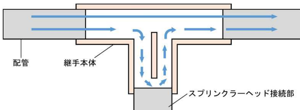
第4-39図 停滞防止継手
