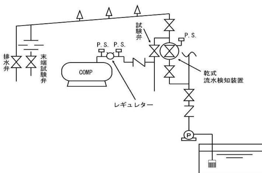
第4-32図 乾式流水検知装置の場合
