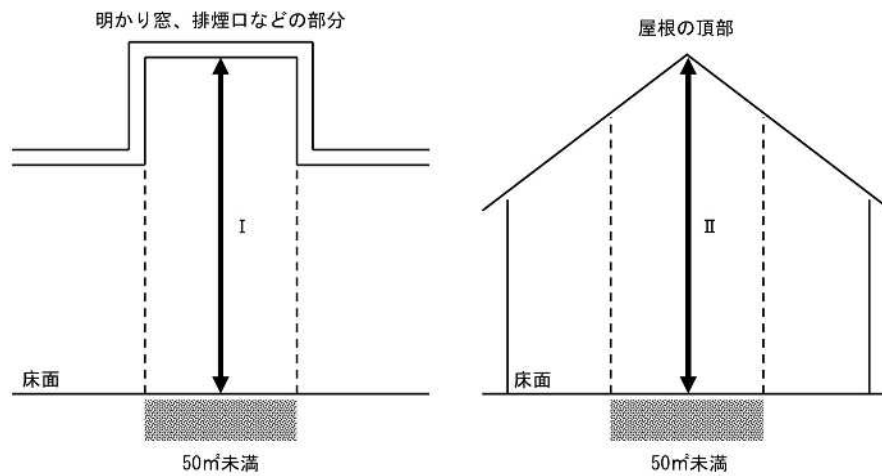
第4-26図（I及びII：6m又は10mを超える部分）
