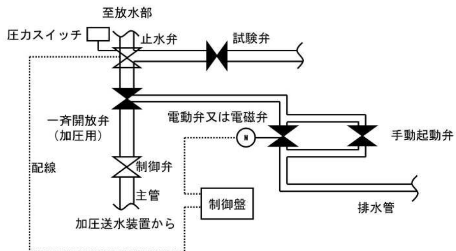
第4-18 図（加圧方式の一斉開放弁等の廻りの配管図例）
