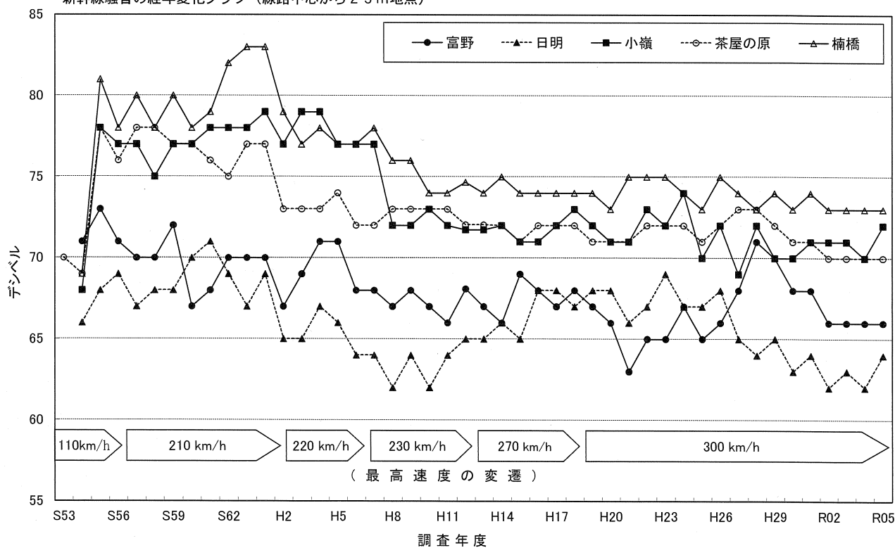
新幹線騒音の経年変化グラフ（線路中心から2.5m地点）
