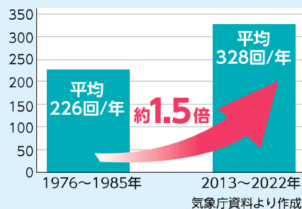
1時間50mm以上の年間大雨の発生回数
