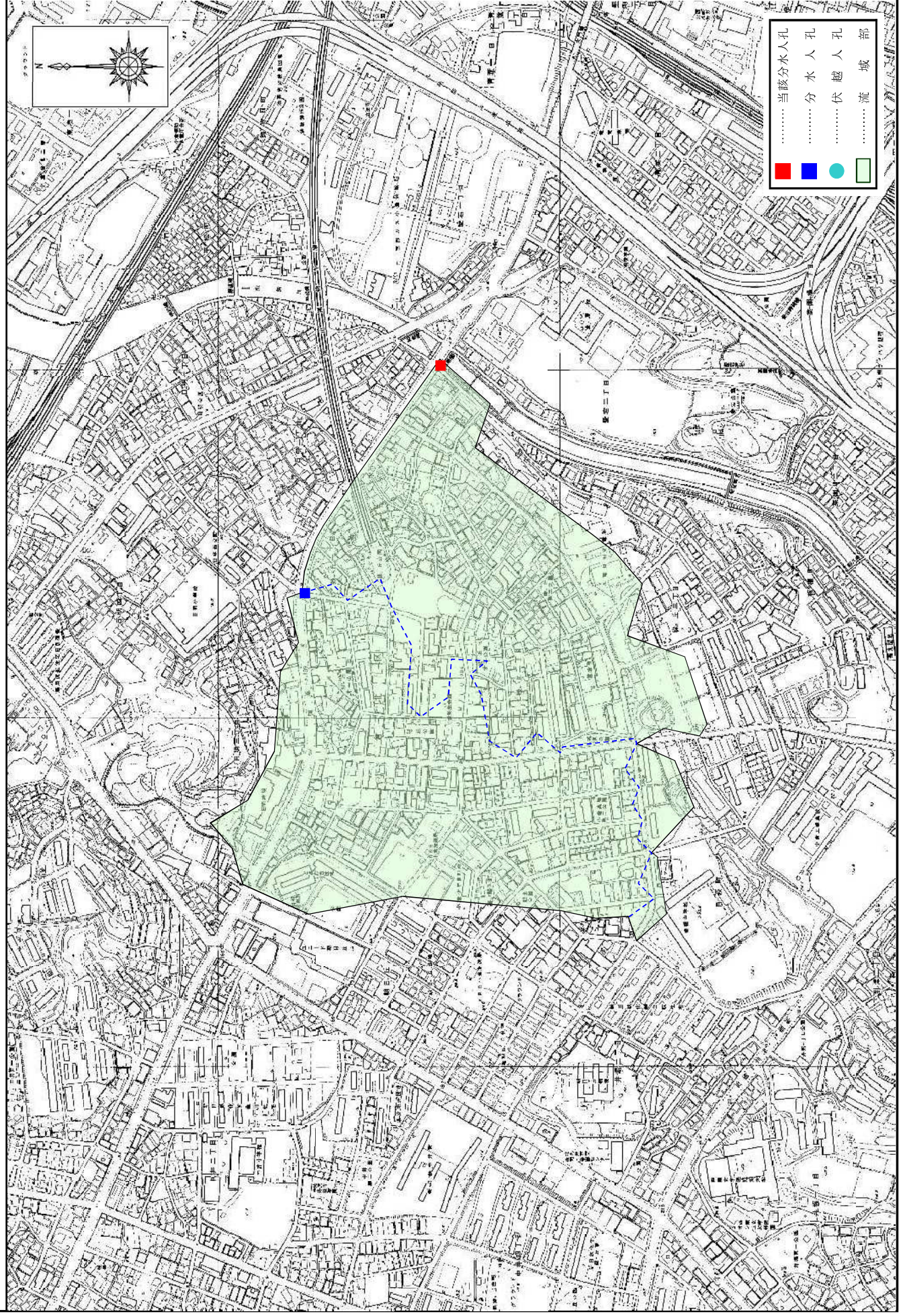
流域図 (B-1) 緑ヶ丘1号 分水人孔 (1)
