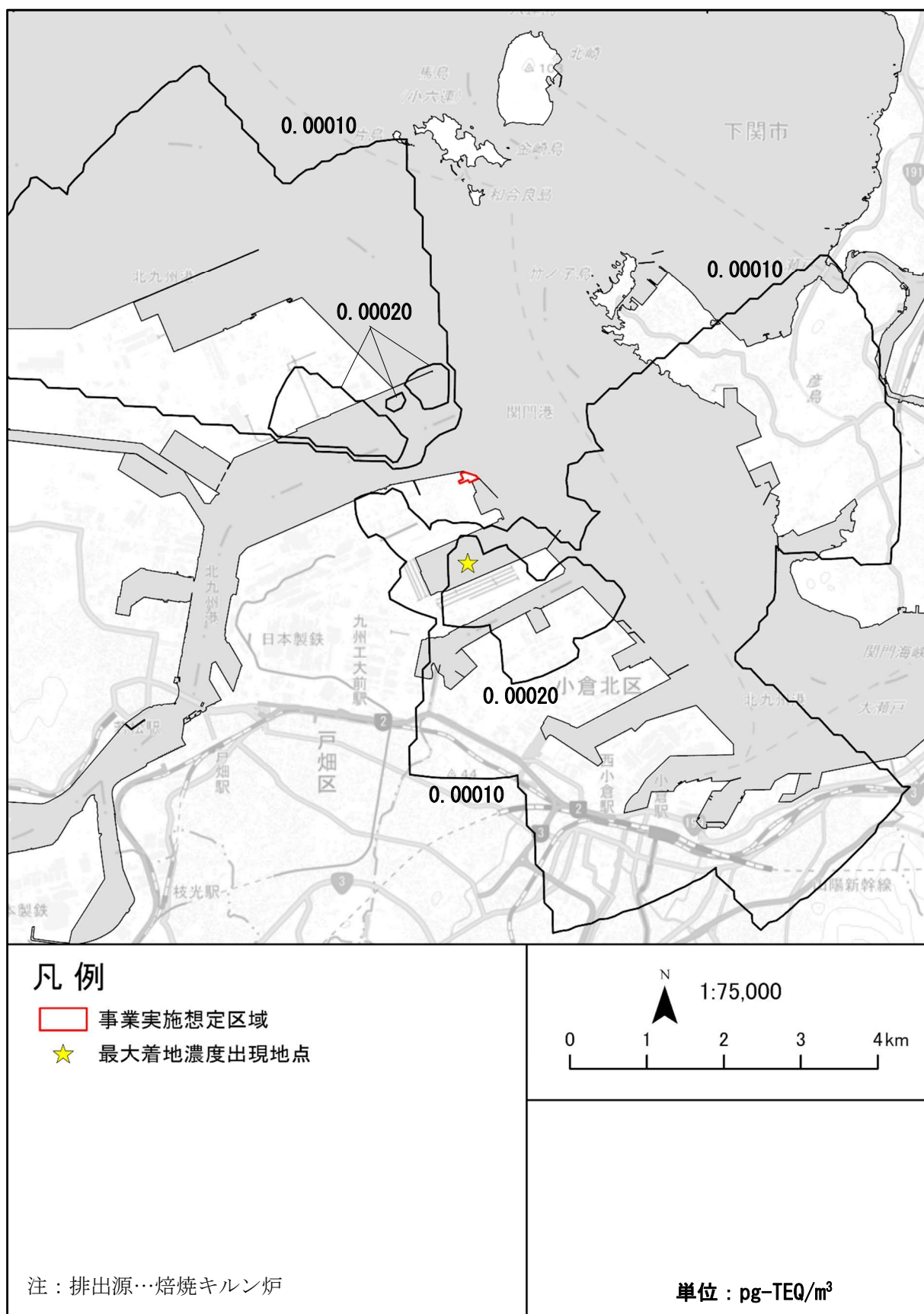
図 4.3-6 (7) 将来の寄与濃度予測結果（ダイオキシン類）：A 案
