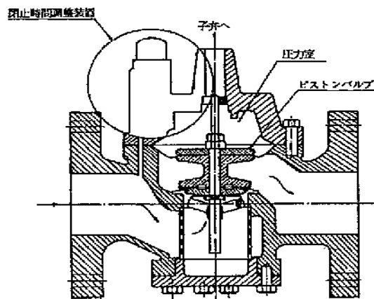
図 6 - 2 1 定水位弁作動の原理
