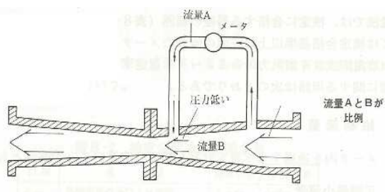
(構造図)
