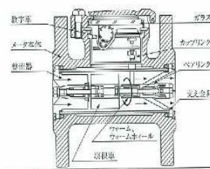
（構造図）
