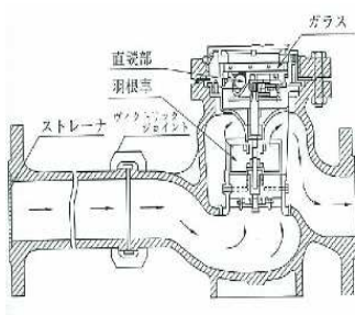
（構造図）
