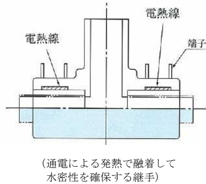
(2) 電気融着式継手
