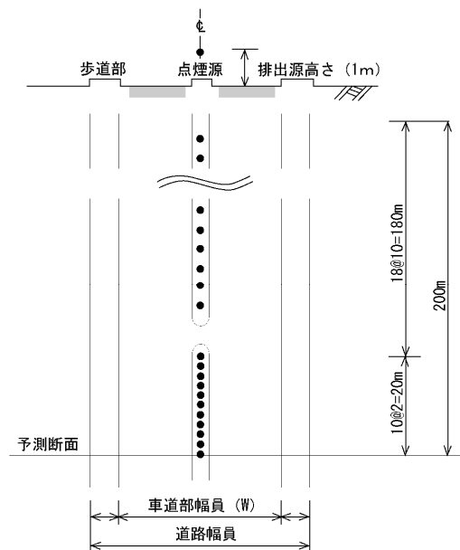
図 11. 1. 1-11 点煙源の配置（一般部）
