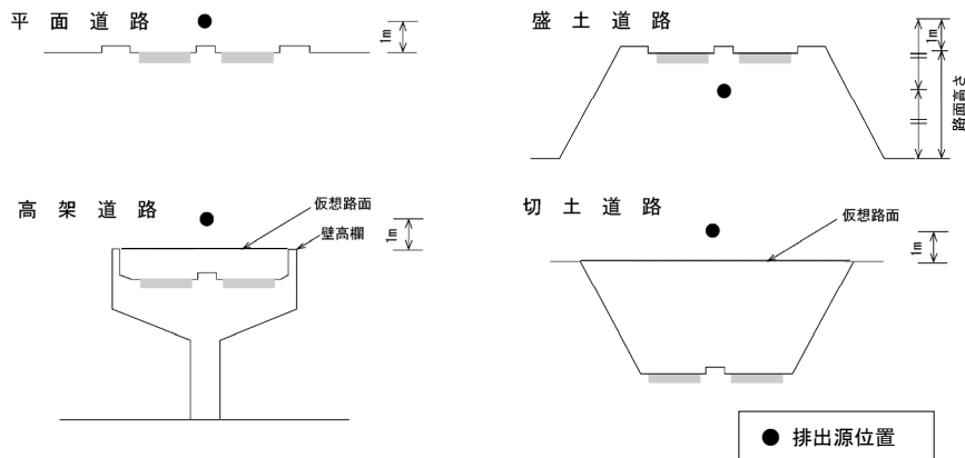
図 11. 1. 1-10 排出源高さの設定
