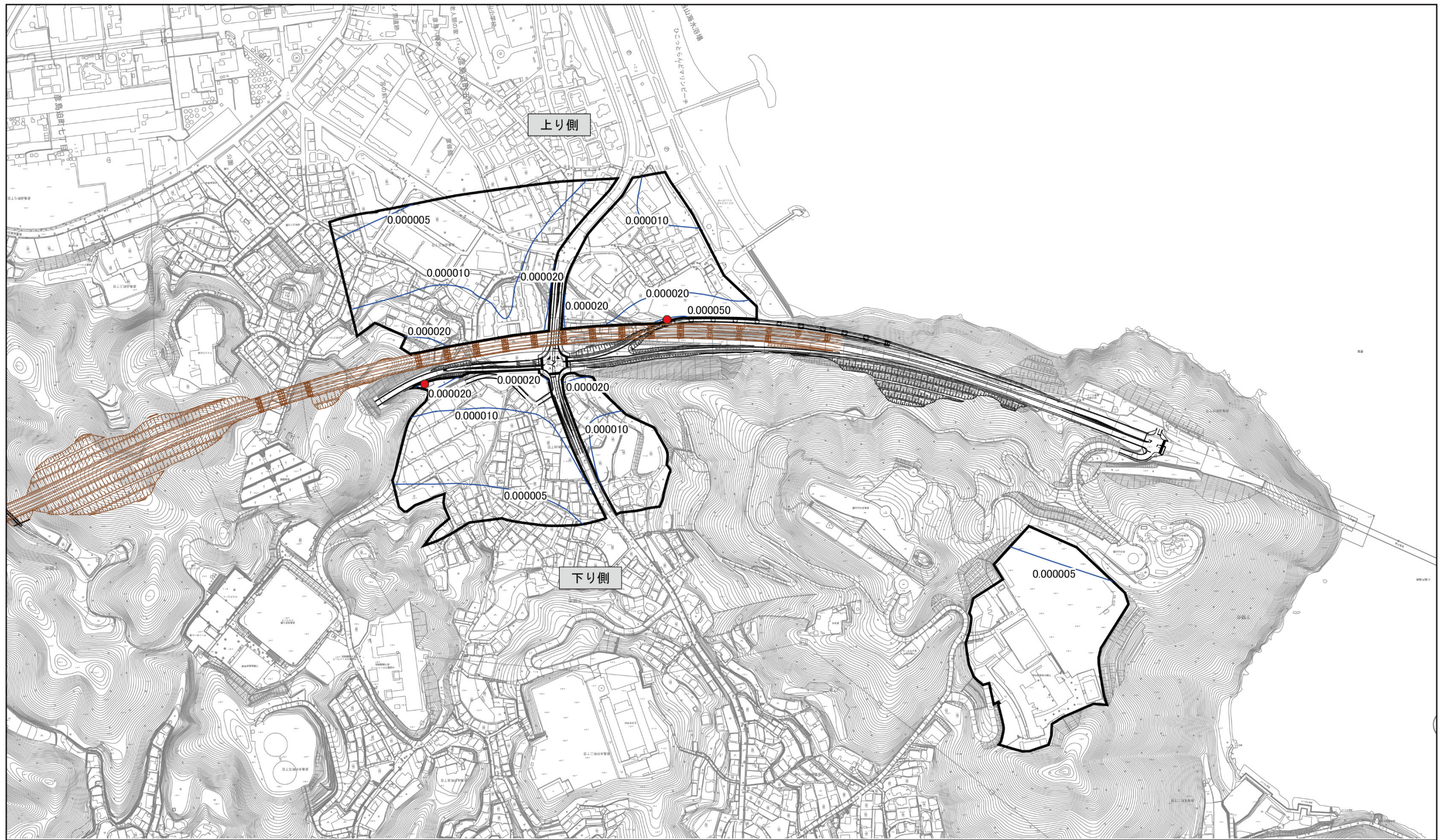
図 11.1.1-16(1) 浮遊粒子状物質の寄与濃度の年平均値の分布状況 (①下関市彦島迫町 6 丁目)
