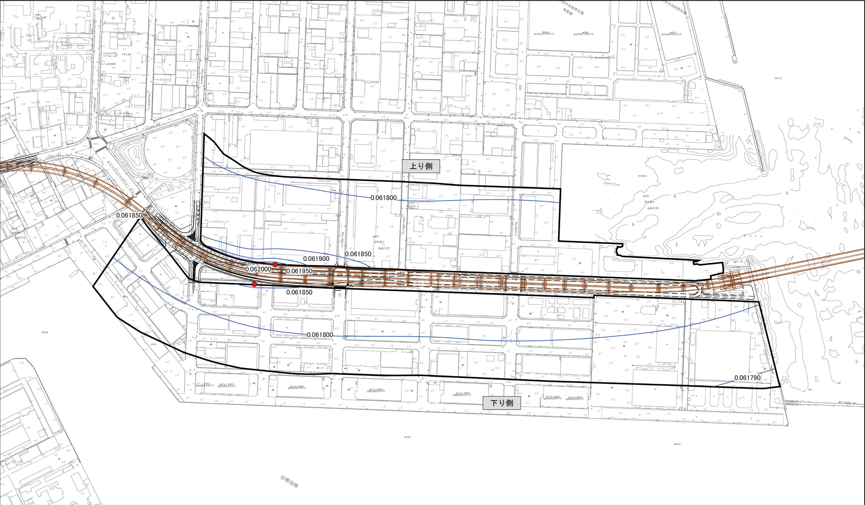
図 11.1.1-17 (3) 浮遊粒子状物質の日 平均値の 2%除外値の分布状況 (㉞北九 州市小倉北区西港町(1)) 凡例 — 対象道路 — 予測地域 ● 予測地点 — 等濃度線 (単位 :mg/m 3 ) 0 50 100 200m 1:5,000
