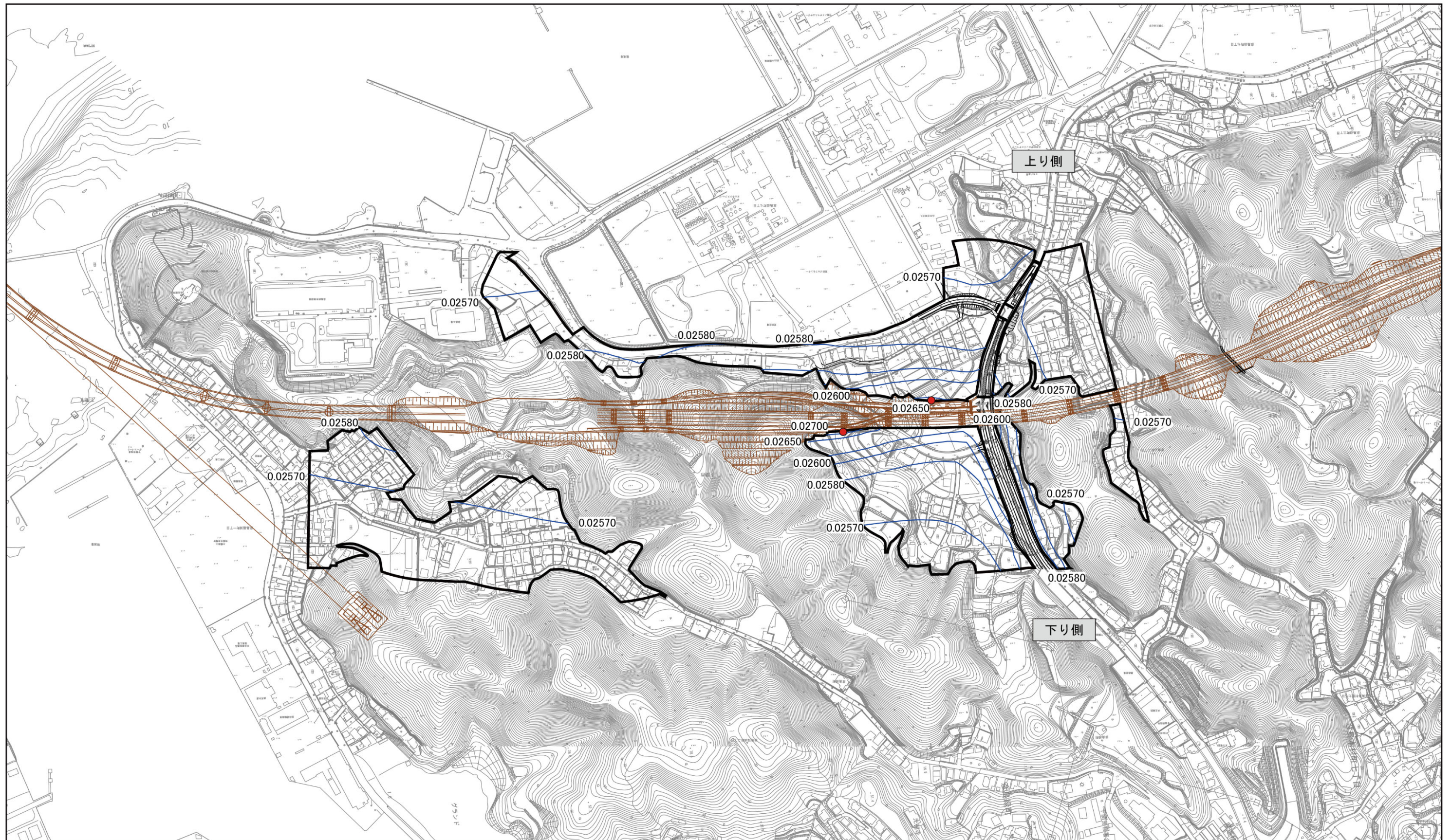
図 11.1.1-15 (2) 二酸化窒素の日平均値の年間 98%値の分布状況 (⑤下関市彦島迫町 1 丁目)
