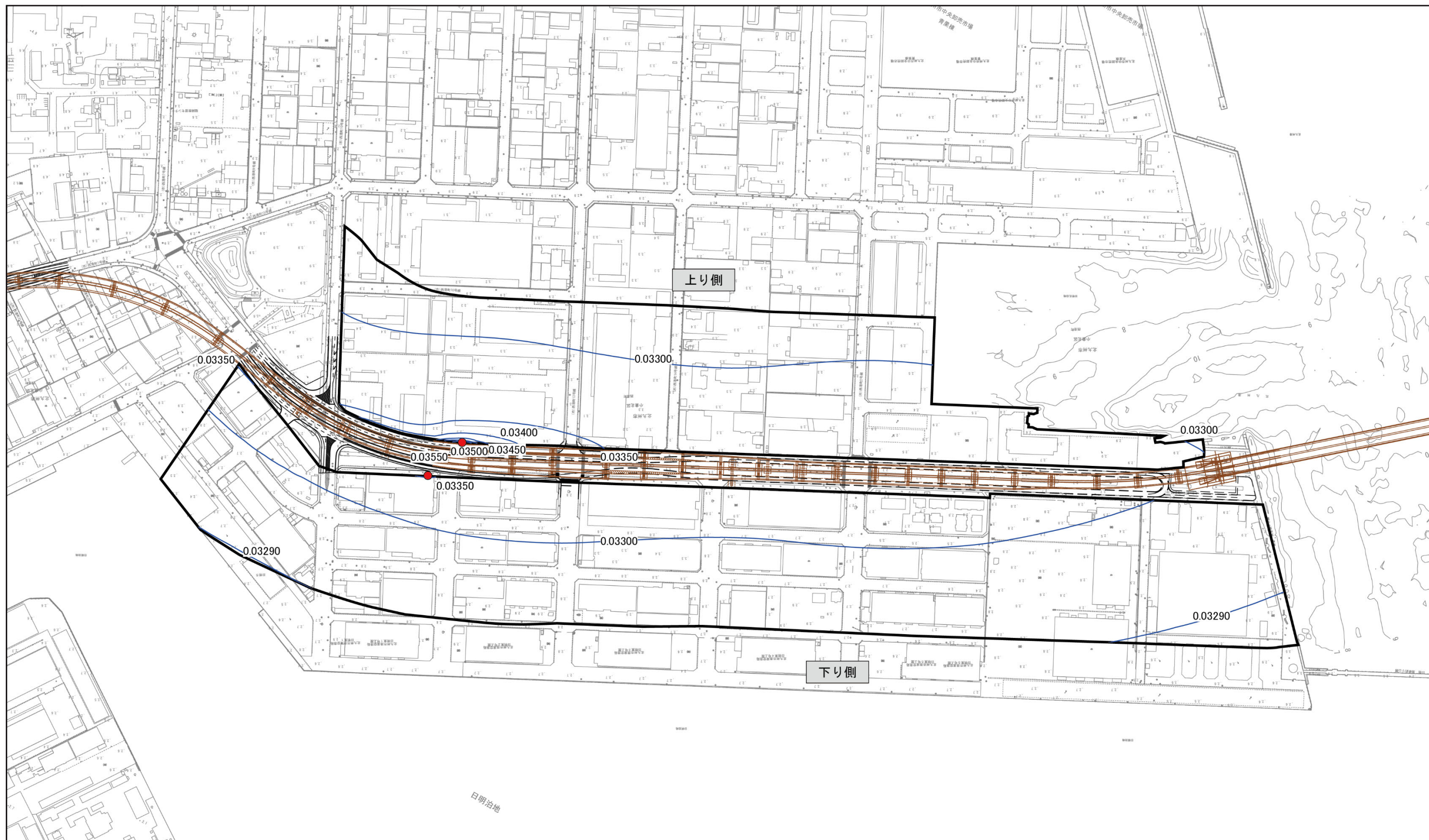
図 11.1.1-15 (3) 二酸化窒素の日平均値の年間 98%値の分布状況 (⑦北九州市小倉北区西港町(1))
