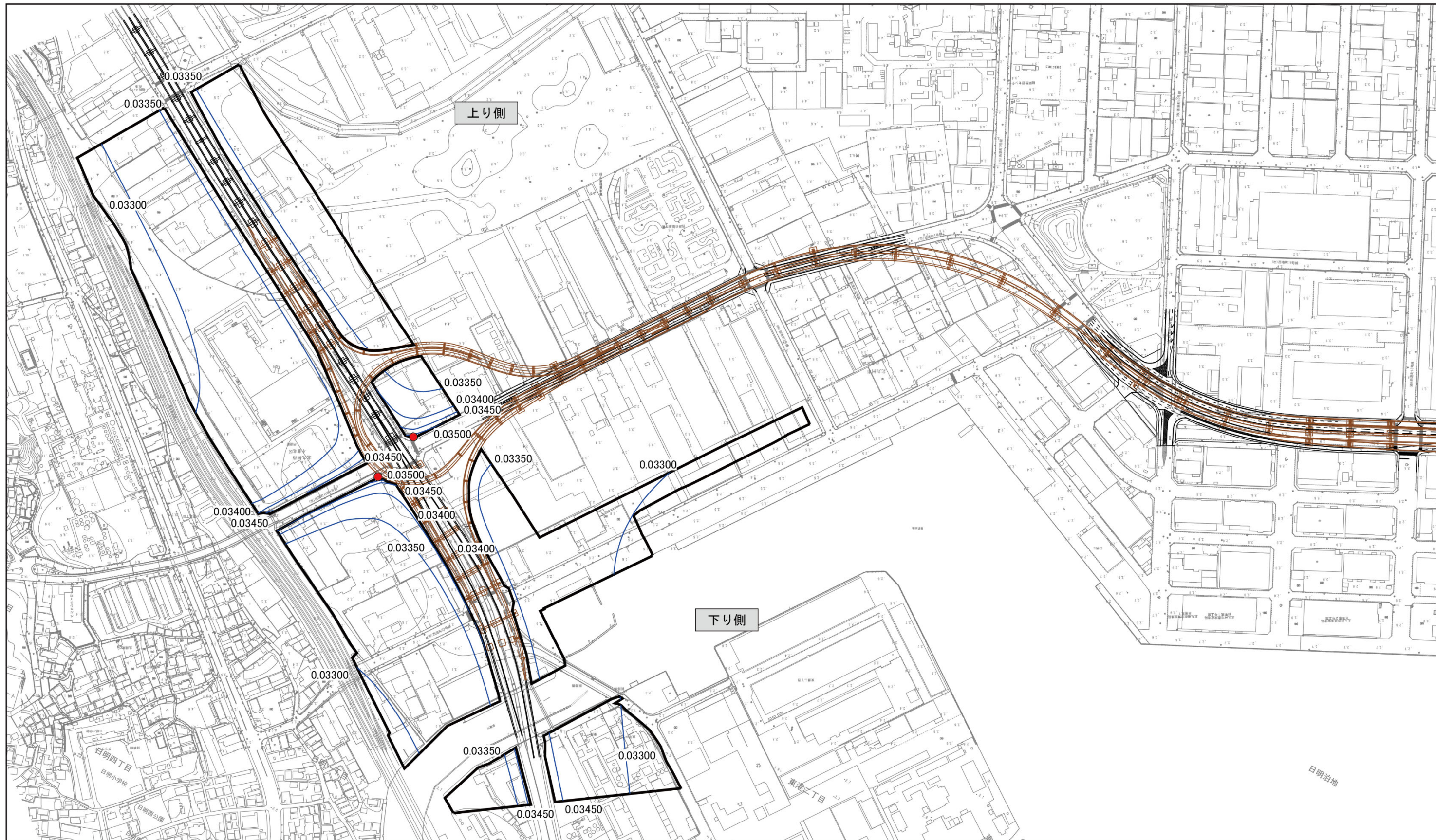
図 11.1.1-15 (4) 二酸化窒素の年平均値の年間 98% 値の分布状況 (⑧北九州市小倉北区西港町(2))
