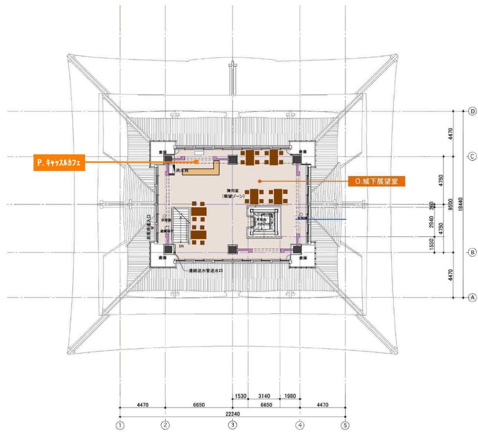
5階平面図 S=1:200
