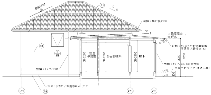
北側立面図・断面図
