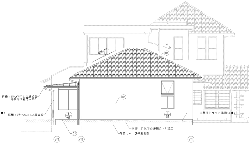
南側立面図
