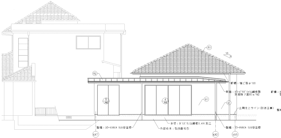
西側立面圖
