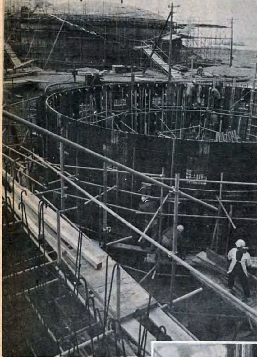
施設の大部分は地下に…地上にそびえるタンクが威容を誇る【消化槽=分離された汚泥を発酵させて減菌する】
