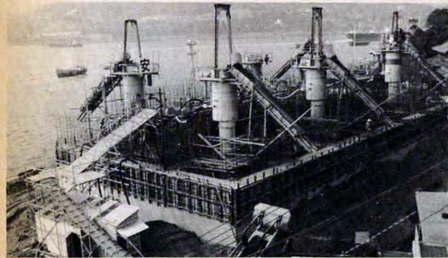
⇒ 早瀬の瀬戸にける関門大橋…いま夢の大橋を受けとめる土台づくりの最中です。コンクリートを積みあげ、その地下を掘り、自分の重みで静かに岩盤にとりつく(ケーソン工法)。48年秋完成し、中国と九州の縦貫自動車道を海上60mの空中で結び本格的なハイウェイ時代をむかえます。
