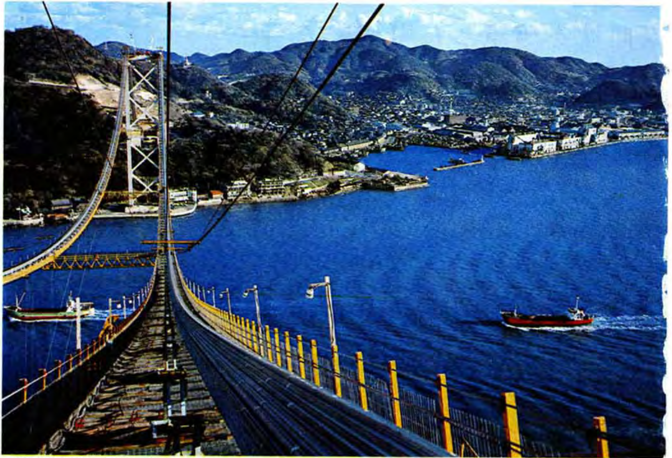
建設中の関門大橋（下関側から）
