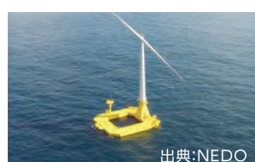
▲響灘沖浮体式洋上風車実証機
