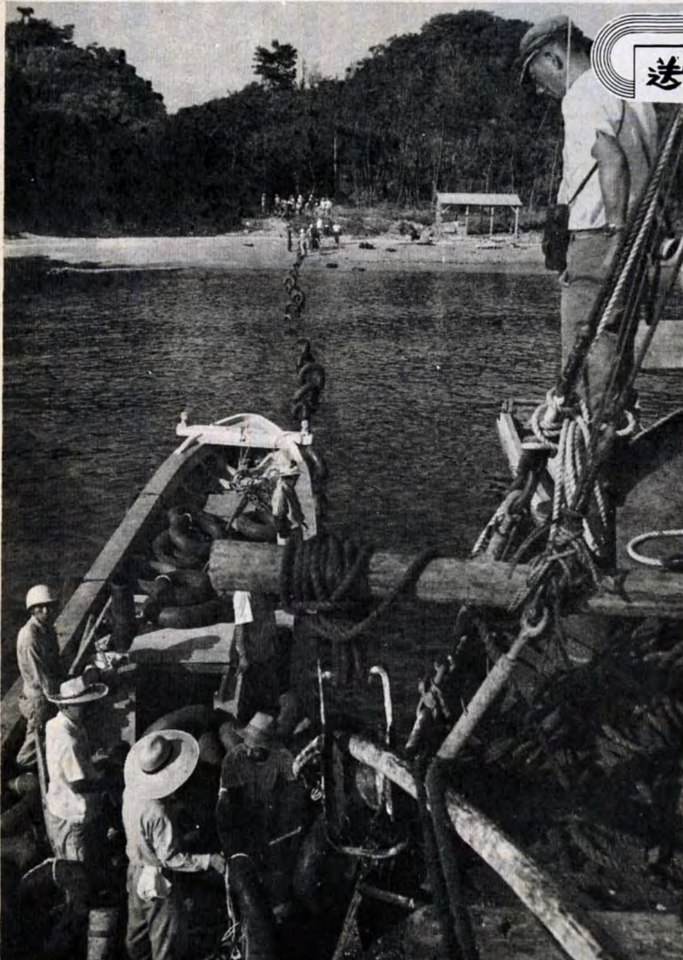
↑藍島から引いてきた4・3キロの海底ケーブルの馬島陸上げ工事
