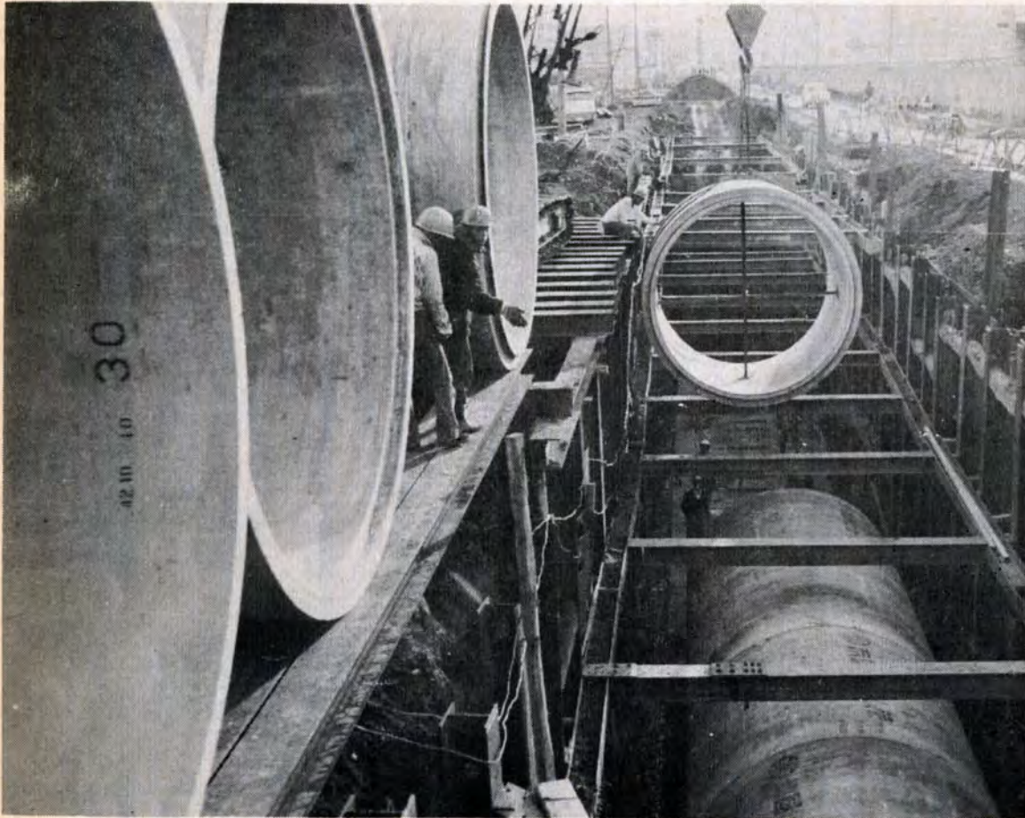
幹線下水道の敷設工事 (小倉区日明埋立地で)
