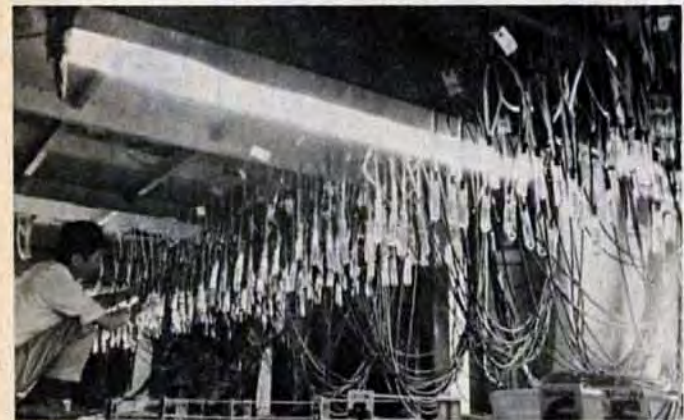
地形模型を作って、風速、風向などいおう酸化物の濃度を調べる風洞実験
