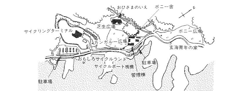
ひびき動物ワールド計画平面図
