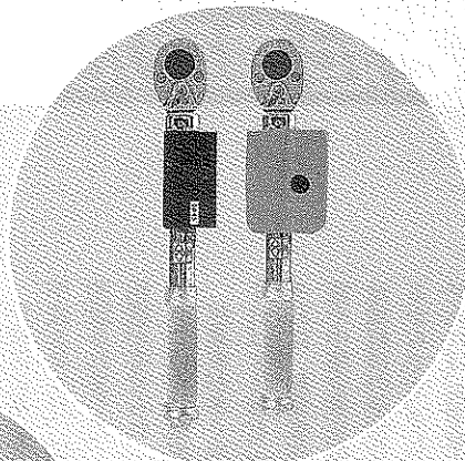
▲内蔵した発信機からの信号で、ネジが決められた力で締められているかどうかを、離れた場所から監視できる機能を備えた「トルクレンチ」。
