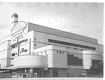
▲「新皇后崎工場」には、ごみ焼却熱を利用した蒸気タービンとガスタービンを組み合わせ、最大3万6300kWを発電する日本で最大のスーパーごみ発電システムが導入されました
